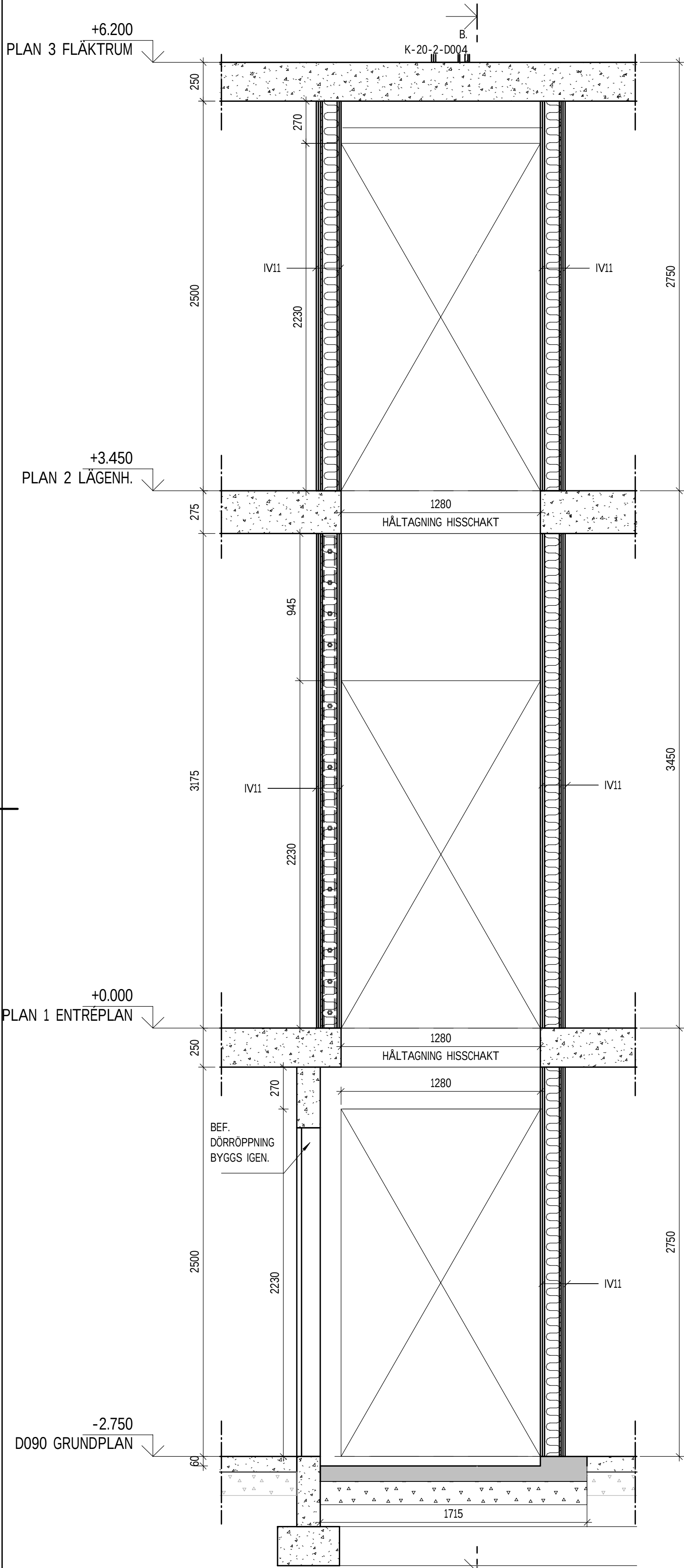
A-A 1 : 20
