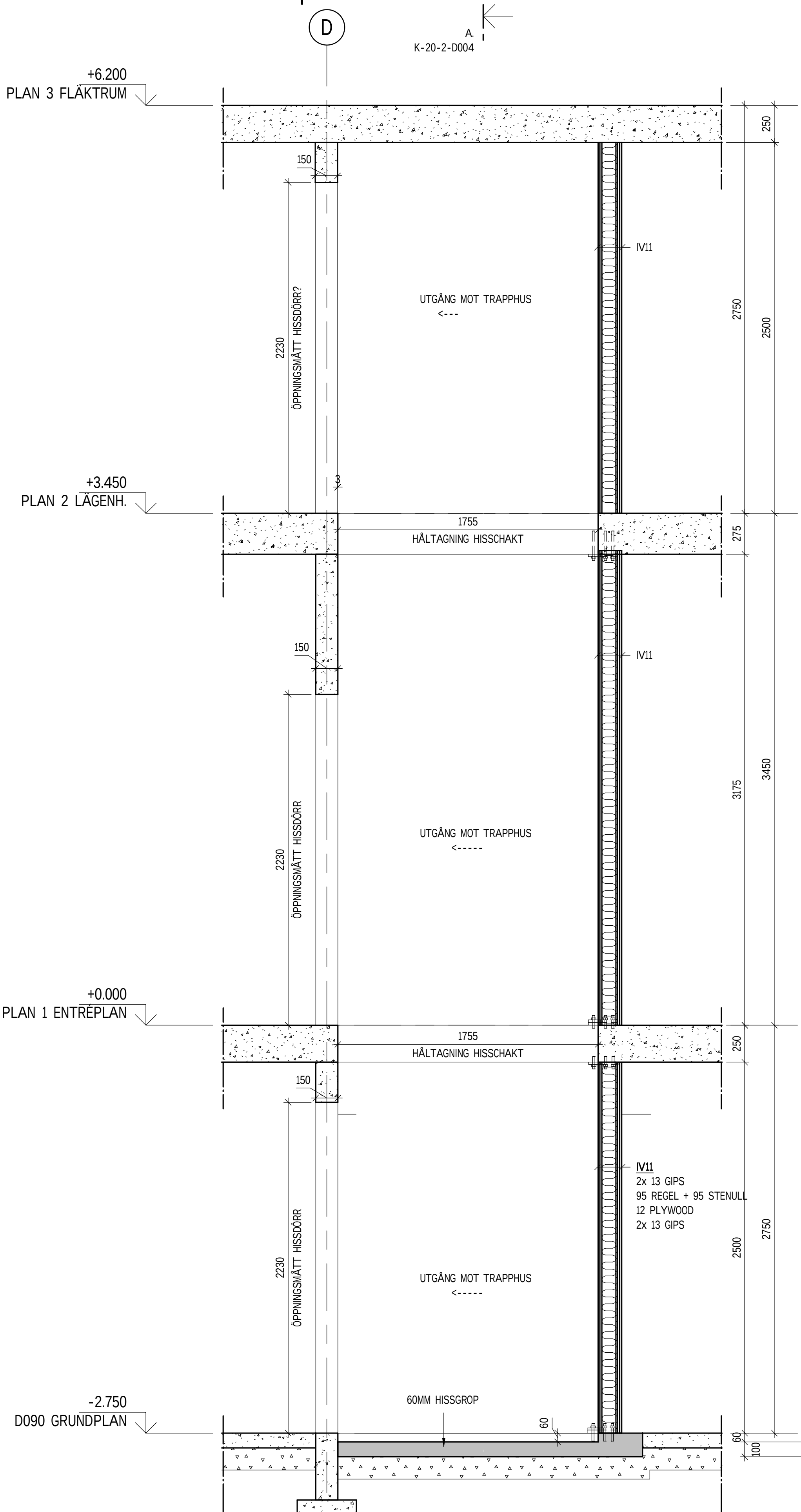
B-B 1 : 20
